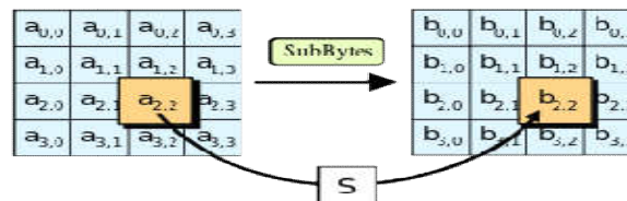
Fig: Sub Byte transformation
