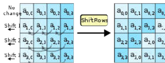
Fig: Shift Rows operation
